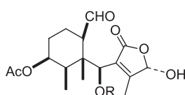
139a R = i But 139b R = Ang
